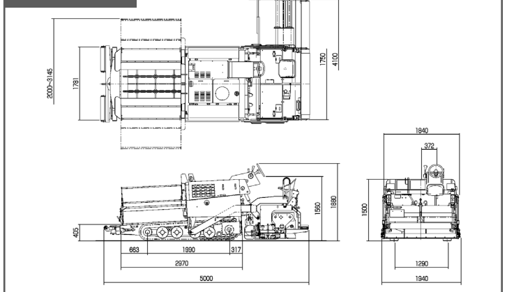
■ 寸法図
